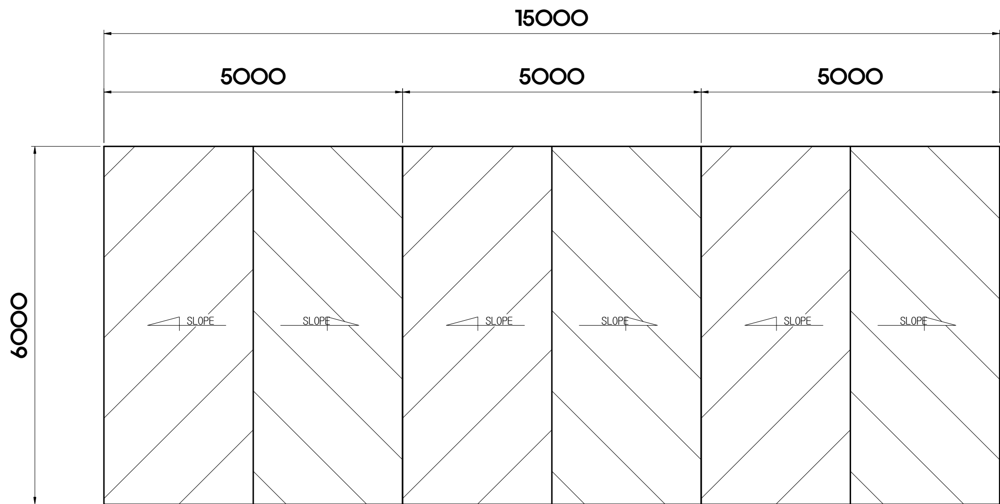
지붕평면도 SCALE=1/60
